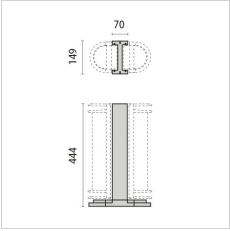
000446 Post 45 H410
